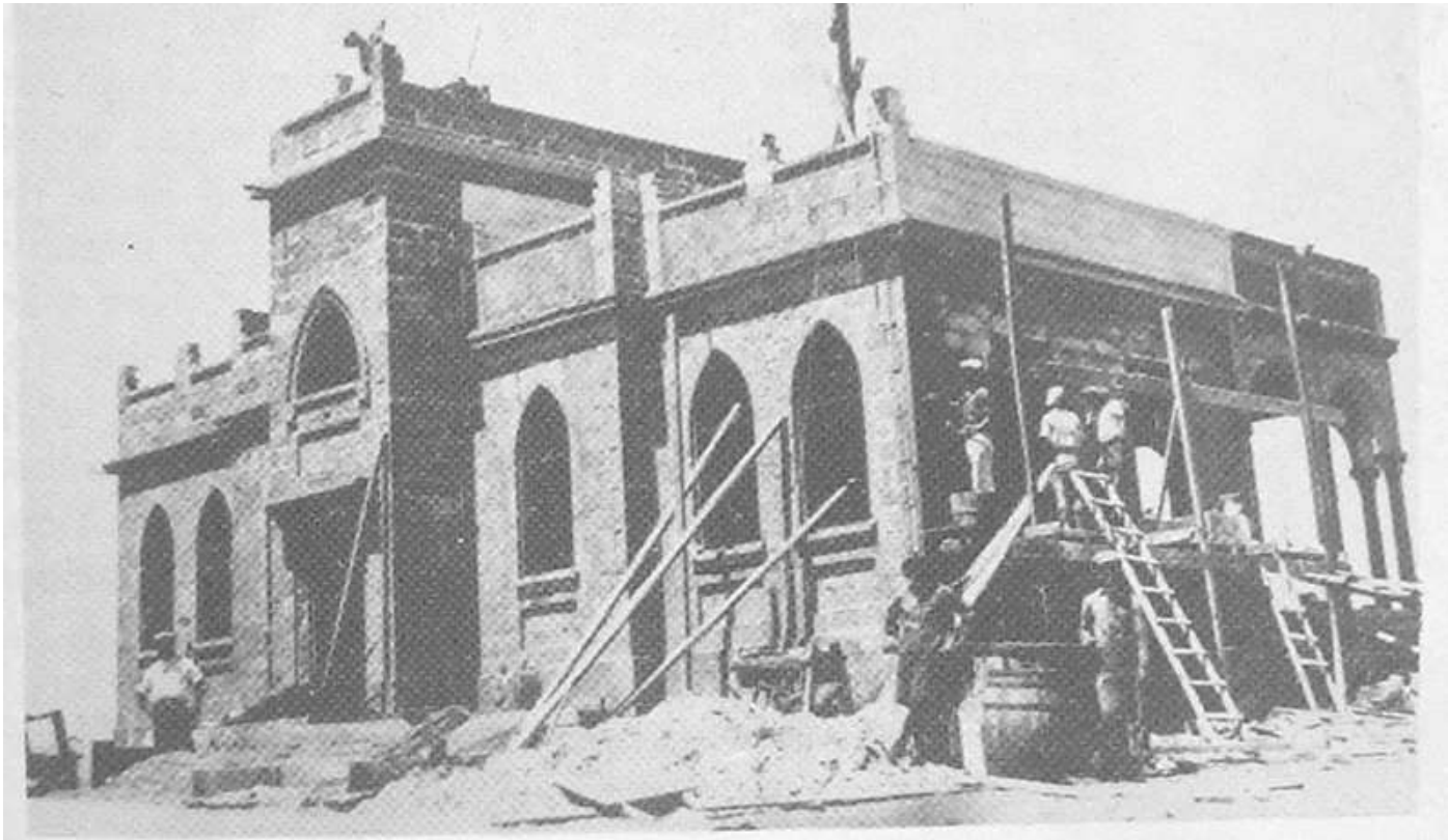
המבנה בבנייתו. בצילום נראים הקירות הנושאים עשויים בלוקים. תשתית הקרניזים העשויה בטון. והשיניות יצוקות מבטון טרומי. מקור: שבעים שנה לכפר סבא.
